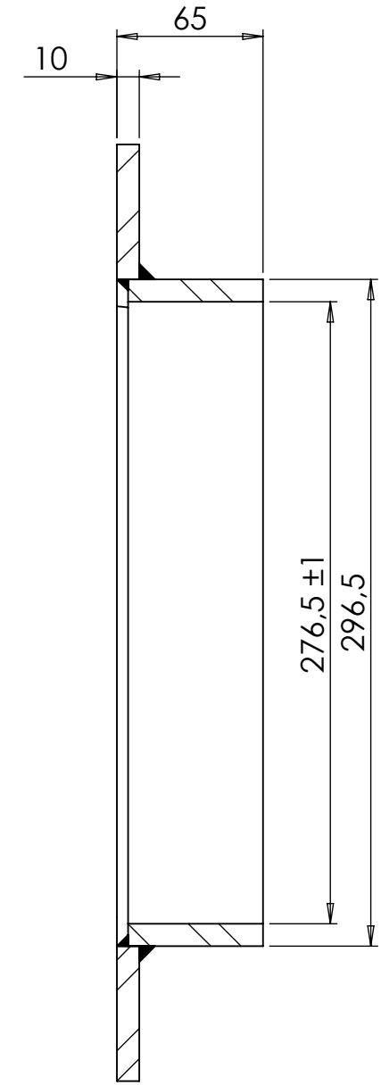
SECTION A-A
