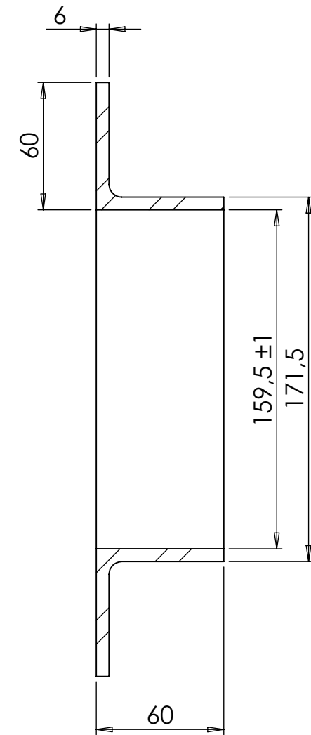
SECTION A-A
