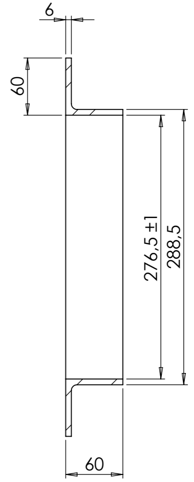
SECTION A-A
