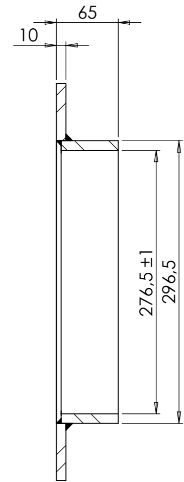
SECTION A-A
