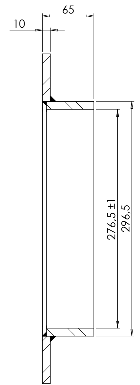
SECTION A-A
