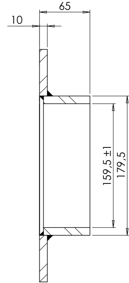
SECTION A-A
