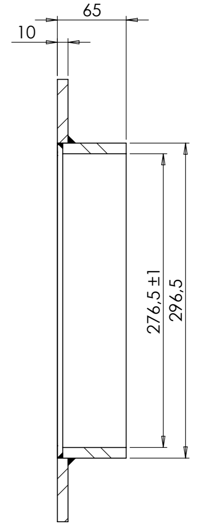
SECTION A-A
