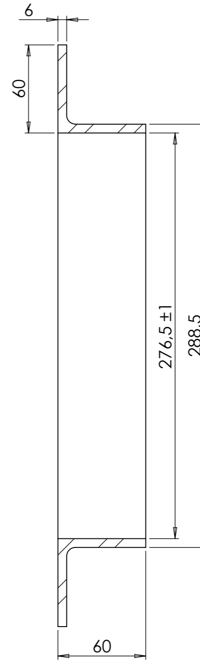
SECTION A-A
