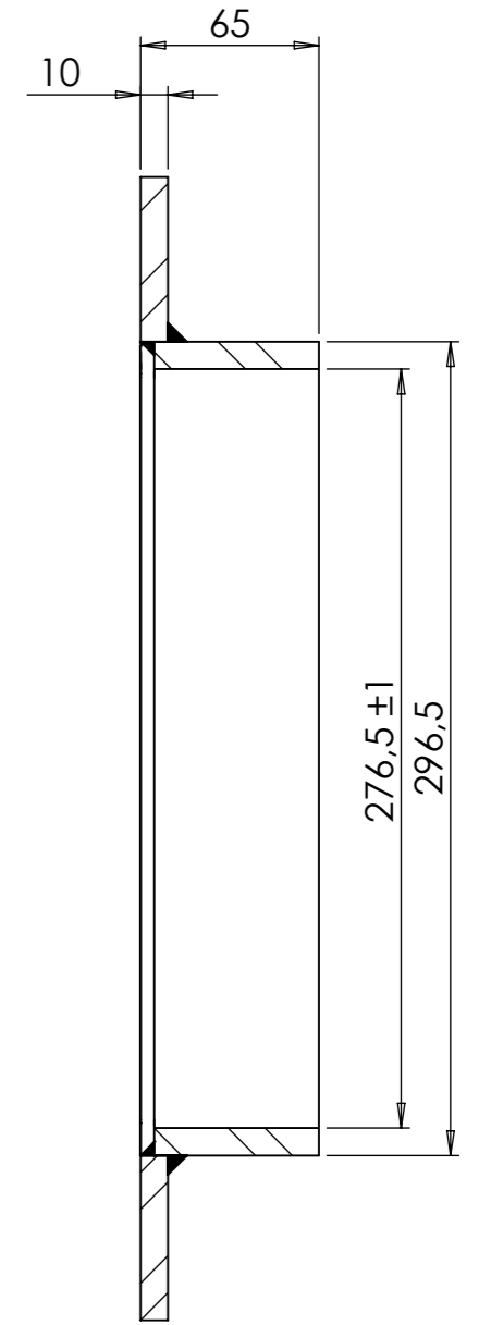
SECTION A-A
