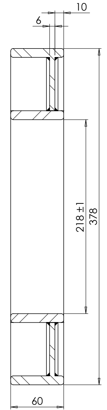
SECTION A-A
