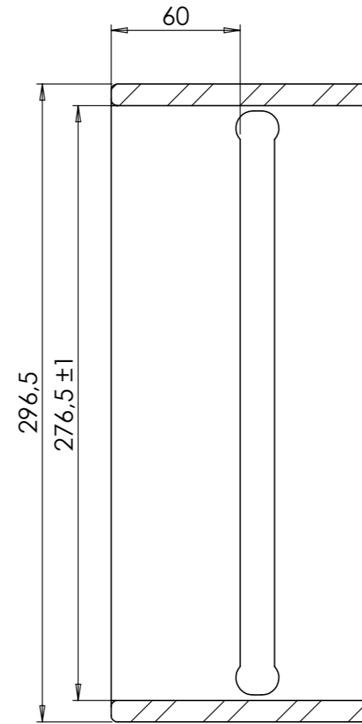
SECTION A-A
